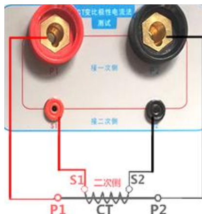
图 13 , CT 变比极性接线图
