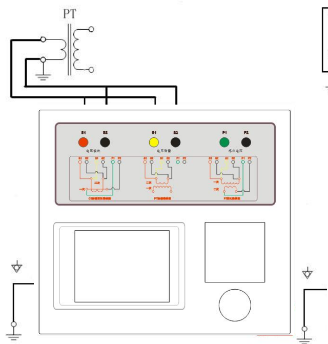
图 2.7 PT 直阻、励磁试验接线方式 第二步：同一 PT 其他绕组开路。
