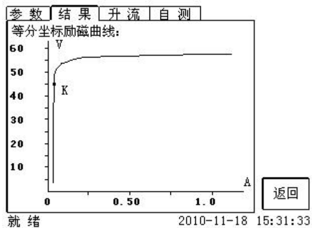
图 2.16 励磁曲线界面
