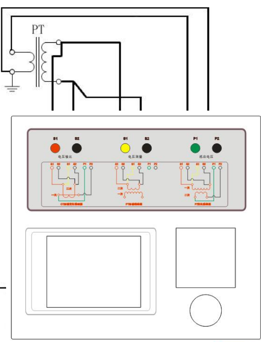
图 2.8 PT 变比、极性试验接线方式
